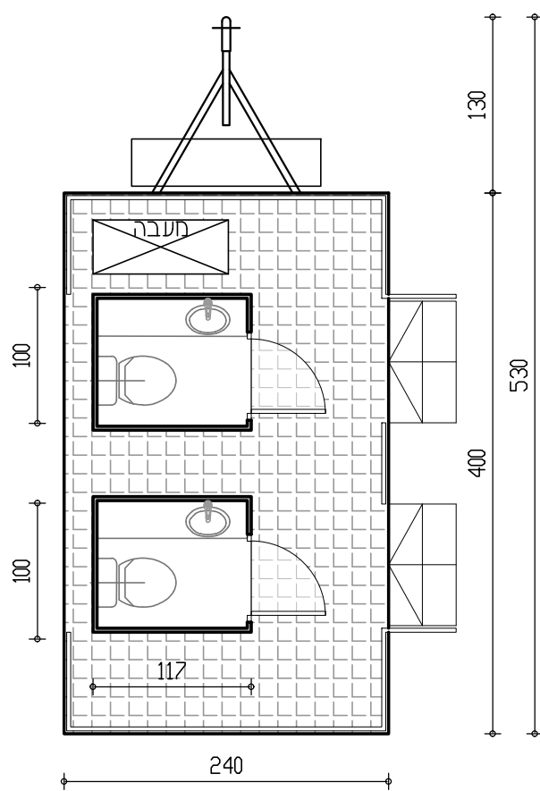
תכנית עגלת שירותים
