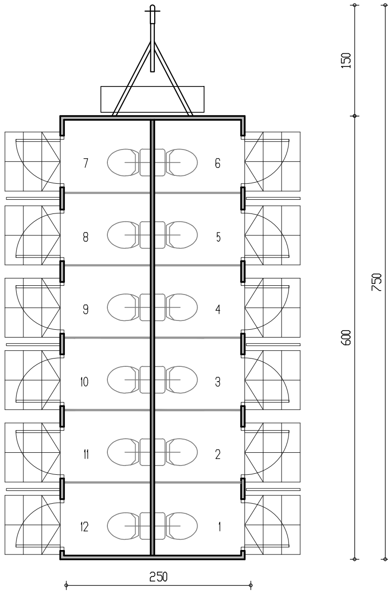
תכנית קרון מעיין 12 תאים
