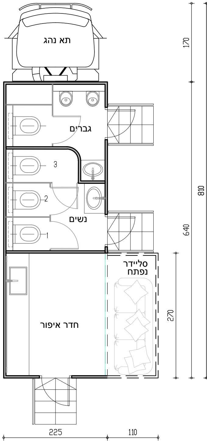
תכנית קרון משאית
